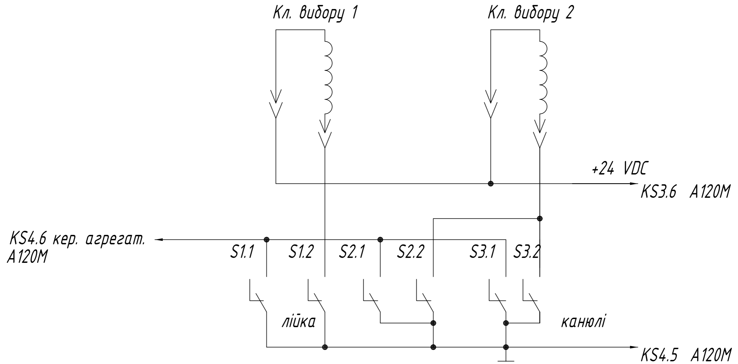
Схема з'єднань для блока асистента установки "ГАЛЛАНТ" автономний (на спареному мікроперемикачеві "DURR")
